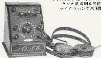
さぐり式鉱石受信機と 両耳レシーバー 初期の大衆用。国産。
